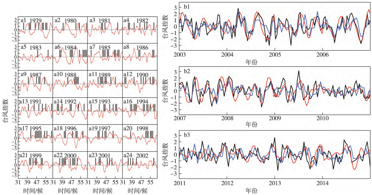
图6 1979—2002年31—61候群发性台风事件(柱状)发生的逐候时间演变及群发性台风指数(红色实线)(a);2003—2014年的观测(黑线)和预报(红色和蓝色为基于两类STPM预报)的群发性台风指数(b)(Zhu et al., 2017)
