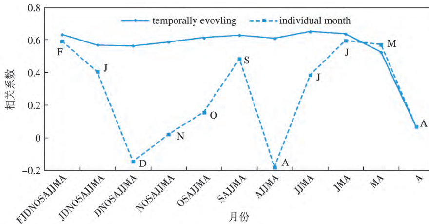
图2 STPM2对台湾地区春雨的时间相关系数预报技巧(实线为采用随时间演变的大尺度预报因子(925 hPa 纬向风)的预报技巧;横轴代表使用的月份信息(例如:JJMA为采用前一年4月演变到7月的大尺度信息);虚线为采用单一月份预报因子(例如:A代表采用4月的大尺度信息)的预报技巧,采用的月份标注在虚线旁)(Hsu et al., 2012)
