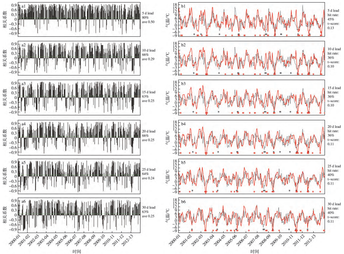
图5 提前5~30 d(a1—a6分别为提前5,10,15,20,25,30 d)预报2000/2001—2012/2013年冬季地表气温的空间相关技巧,即预报场与实际观测的EOF前三模态组合场的空间相关系数(a;绿线为置信度99%的显著性检验);提前5~30 d(b1—b6分别为提前5,10,15,20,25,30 d)预报(红线)与观测(黑线)的南京站地表气温及其极端冷事件(b;预报为红色方框,观测为黑色方框;图右标注预报命中百分比和预报风险评分)(Zhu and Li, 2017c)
