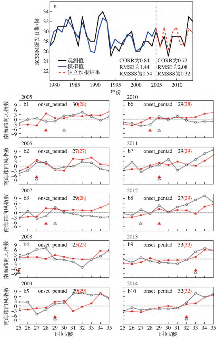
图7 基于PEM的南海季风爆发日期序列(1979—2014年)(a;黑色为观测,蓝色为模拟结果,红色为独立预报结果);基于STPM预报南海季风爆发期间(25—35候)的南海地区纬向风指数(b;黑线为观测,红线为预报,黑三角为观测爆发日期,红三角为预报观测日期)(Zhu and Li, 2017b)
