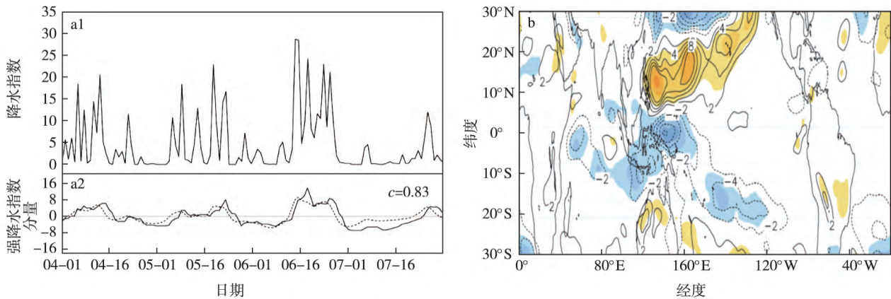
图3 2010年4—7月福建强降水指数时间序列及通过非传统带通滤波(实线)和 Butterworth 带通滤波(虚线)的10~60 d 强降水指数分量(a; 相关系数0.83); 2013年12月1日的10~60 d 850 hPa 纬向风场(b, 单位: \text{m} \cdot \text{s}^{-1} ; 阴影和等值线分别为带通滤波和非传统带通滤波提取的信号)(Hsu et al. 2015)
