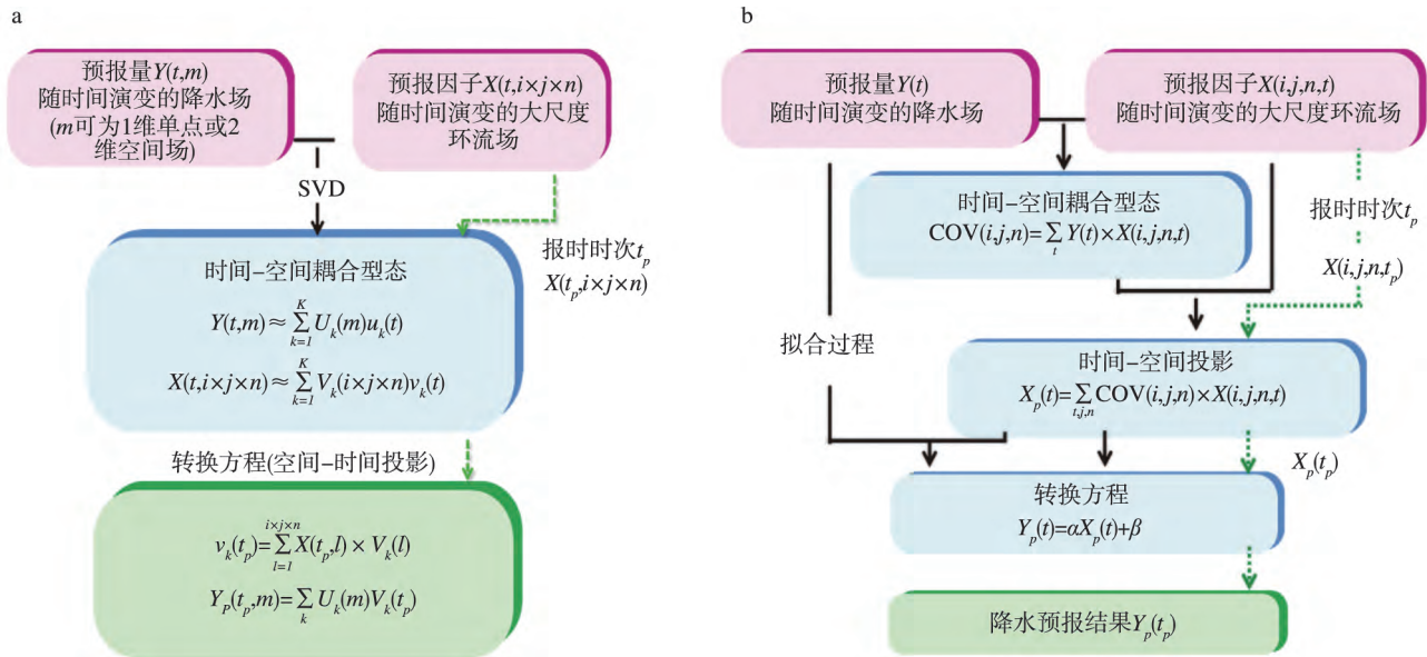
图1 两种STPM预报的主要步骤(STPM1预报模型是基于SVD分析来提取预报量和预报因子的时间-空间耦合信息特征,并建立预报方程( X 和 Y 分别为标准化的大尺度预报因子和预报量, i 和 j 为空间格点, t 为时间, n(m) 分别为 t 之前(之后)的超前(滞后)候, K 为所取的前 K 个的SVD模态, U_k 和 V_k 为预报量和预报因子的奇异向量, u_k 和 v_k 则为对应的时间系数;黑色实线箭头代表建模流程,绿色虚线箭头为 t_p 时次的预报流程。STPM2类似STPM1,但预报模型是基于斜方差(covariance,COV)来提取预报量和预报因子的时间-空间耦合模态, X_p 为大尺度预报因子对COV的投影,再利用多元线性回归建立转换/预报方程。详细步骤及说明请见参考文献Hsu et al.(2012)及Hsu et al.(2015): (a) STPM1; (b) STPM2
