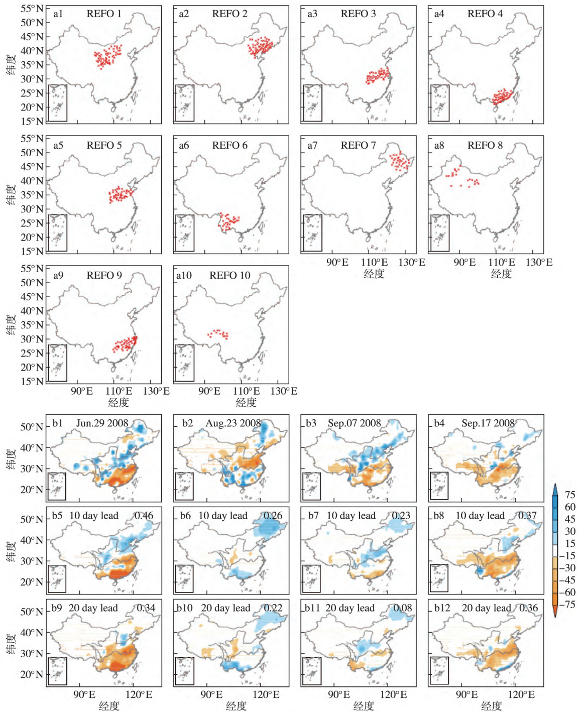
图4 1979—2010年中国夏季季节内(10~80 d)降水的REOF前十个模态(a;红色标记载荷值超过0.4的站点);2008年夏季预报实例(b;由上、中、下列分别是观测、提前10 d、20 d预报的降水异常;蓝色和橘红色阴影分别为降水正异常和负异常;单位: 0.1 \text{ mm} \cdot \text{d}^{-1} ;右上角标注空间相关系数)(Zhu and Li 2017b)
